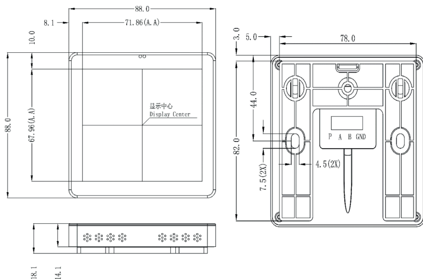
Габариты пульта:
