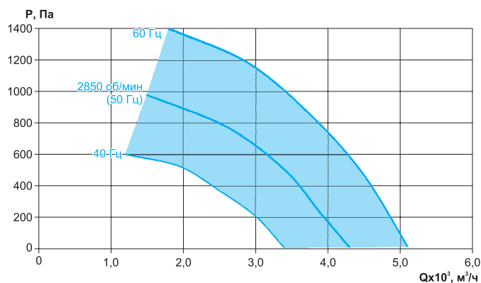
ВРС-К-80-50/31-РК635-1,5/3000/220-380
