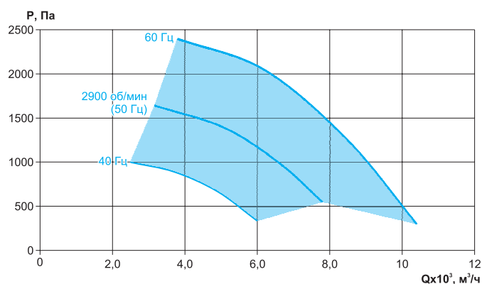
ВРС-К-80-50/40-РК635-5,5/3000/220-380
