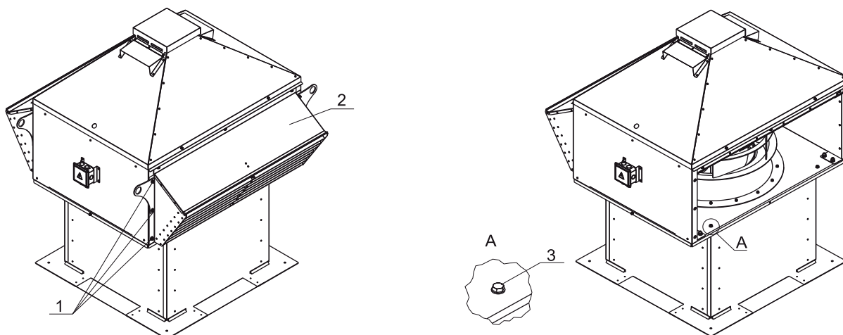
Рисунок 5.3 – Монтаж РОКС-ВКРС
